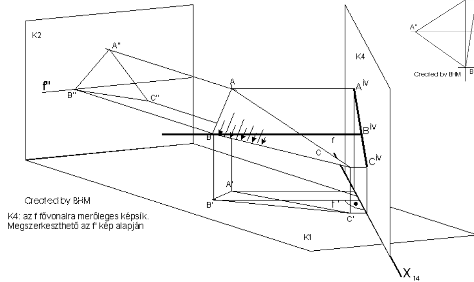
A szerkesztés lépései papíron vetületi ábrázolásnál. Előzmény: 3. - 4. kép szerkesztése
