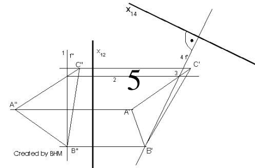
A szerkesztés lépései papíron vetületi ábrázolásnál. Előzmény: 3. - 4. kép szerkesztése
