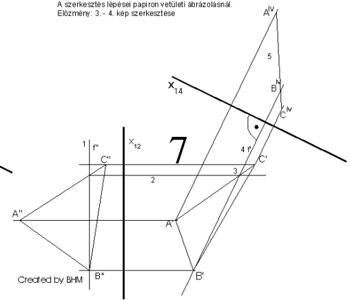
A szerkesztés lépései papíron vetületi ábrázolásnál. Előzmény: 3. - 4. kép szerkesztése
